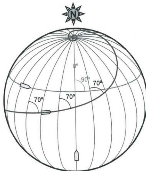
Loxodrómia descrita, navegando ao Rumo (R) de 070^\circ .
